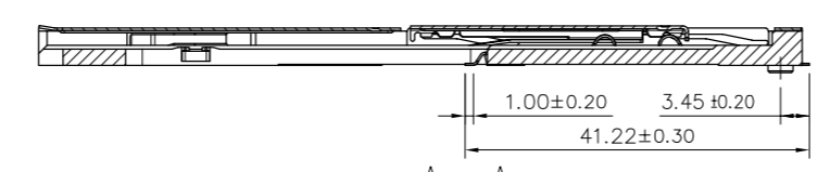
SECTION A-A SCALE 1:1
